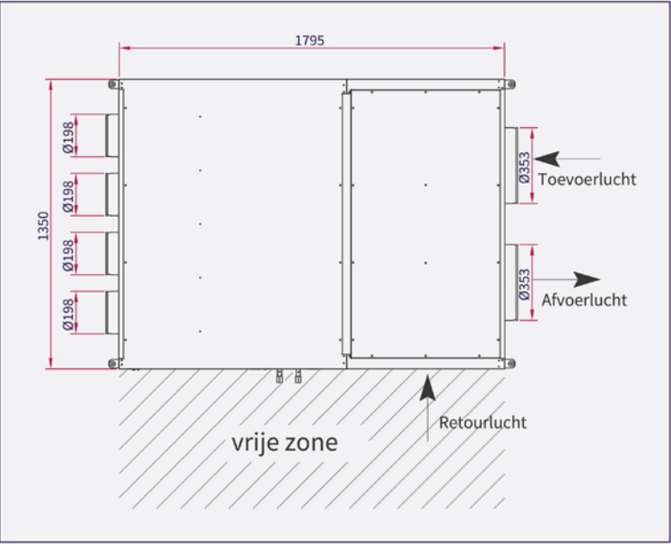
CP16.30 H-S (gespiegelde uitvoering) - bovenaanzicht
