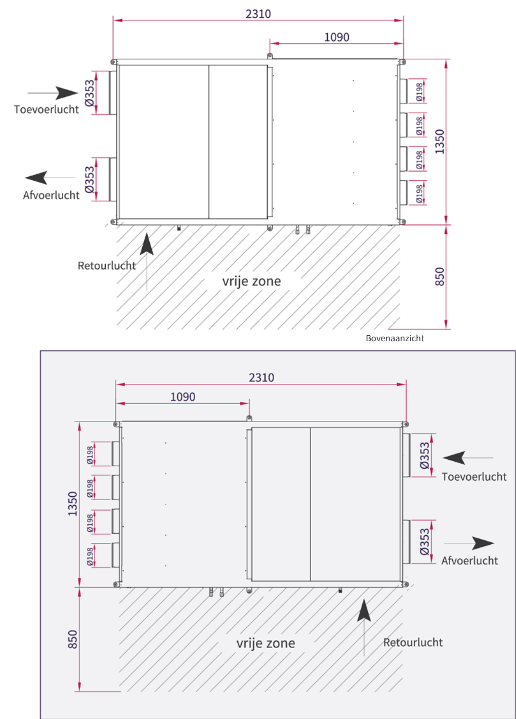
CP14.30 H-S (gespiegelde uitvoering) - bovenaanzicht
