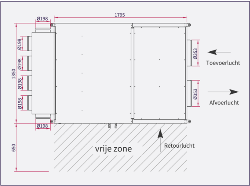
CP20.30 H-S (gespiegelde uitvoering) - bovenaanzicht
