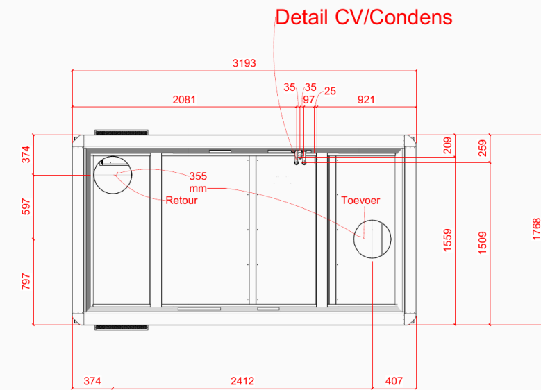
2 3D - W57_Lucht Onderaanzicht
