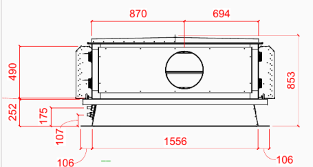
7 Rechter Zijaanzicht 1 : 20
