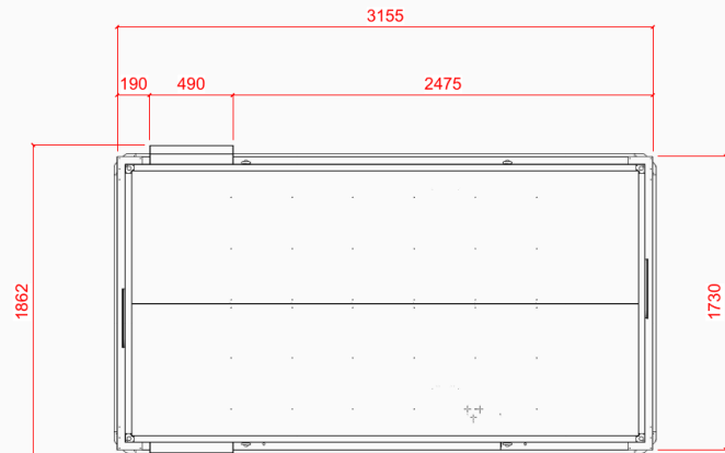
1 3D - W57_Lucht Bovenaanzicht
