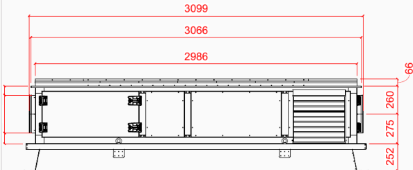
5 Achter Aanzicht 1 : 20
