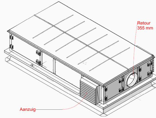
4 3D Vooraanzicht
