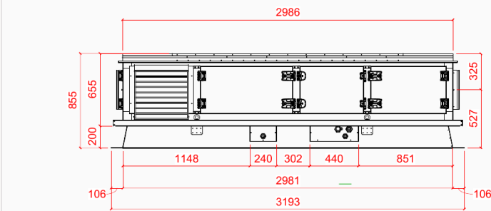
8 Voor Aanzicht 1 : 20
